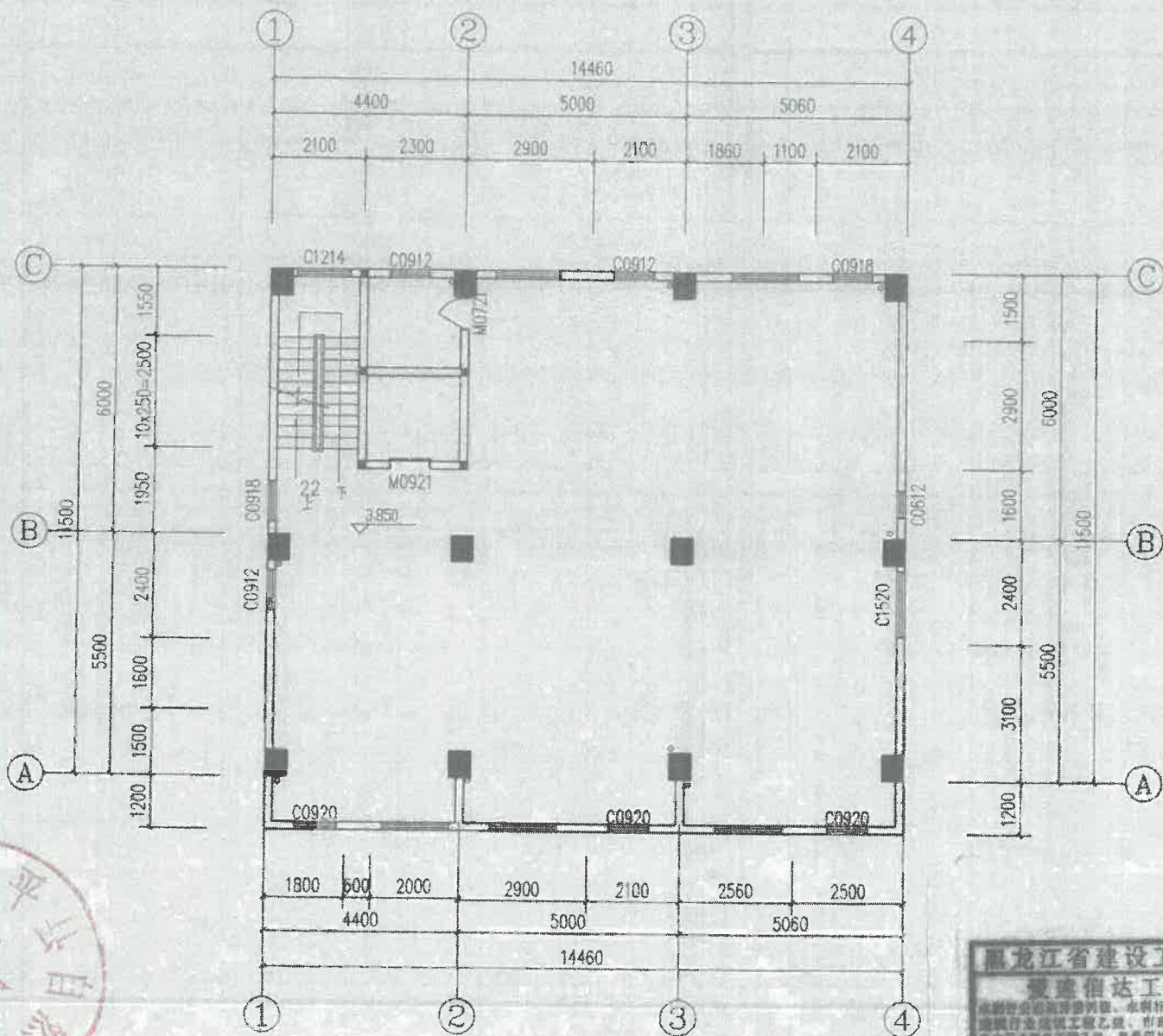
二层平面图 1:100
