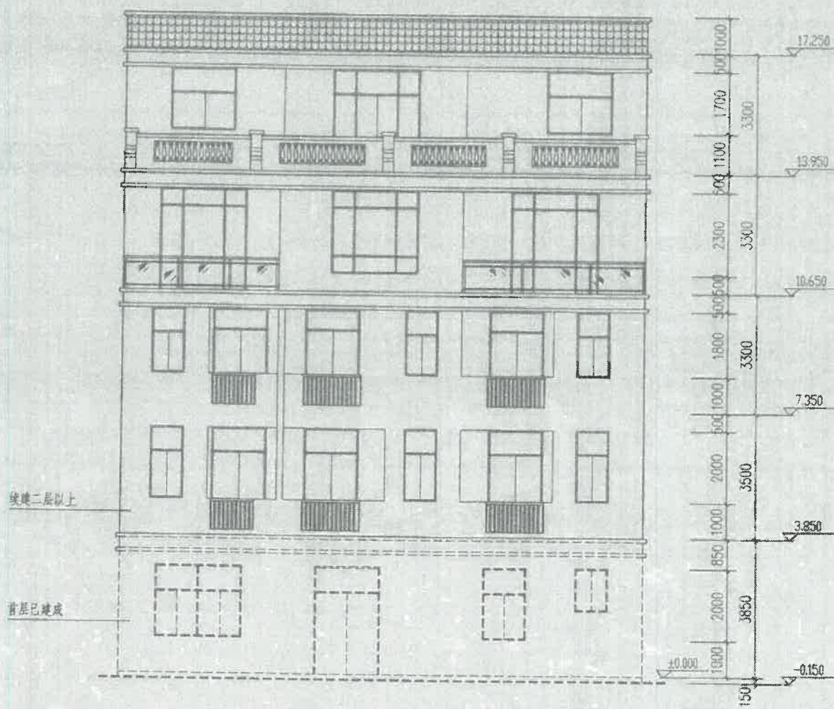
正立面图 1:100
