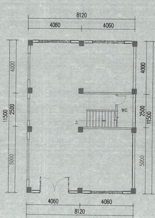
一层平面图
