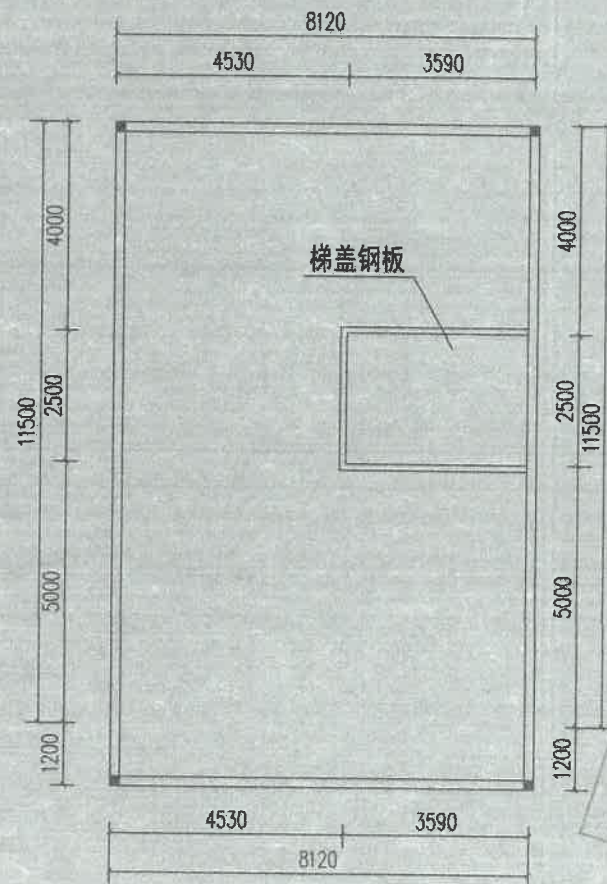
天面平面图
