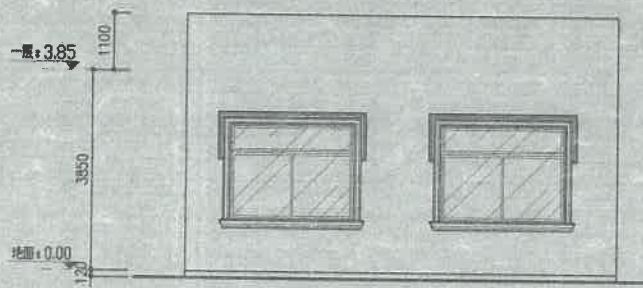
背立面图
