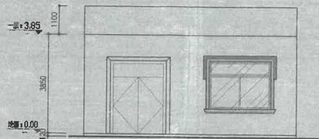
正立面图
