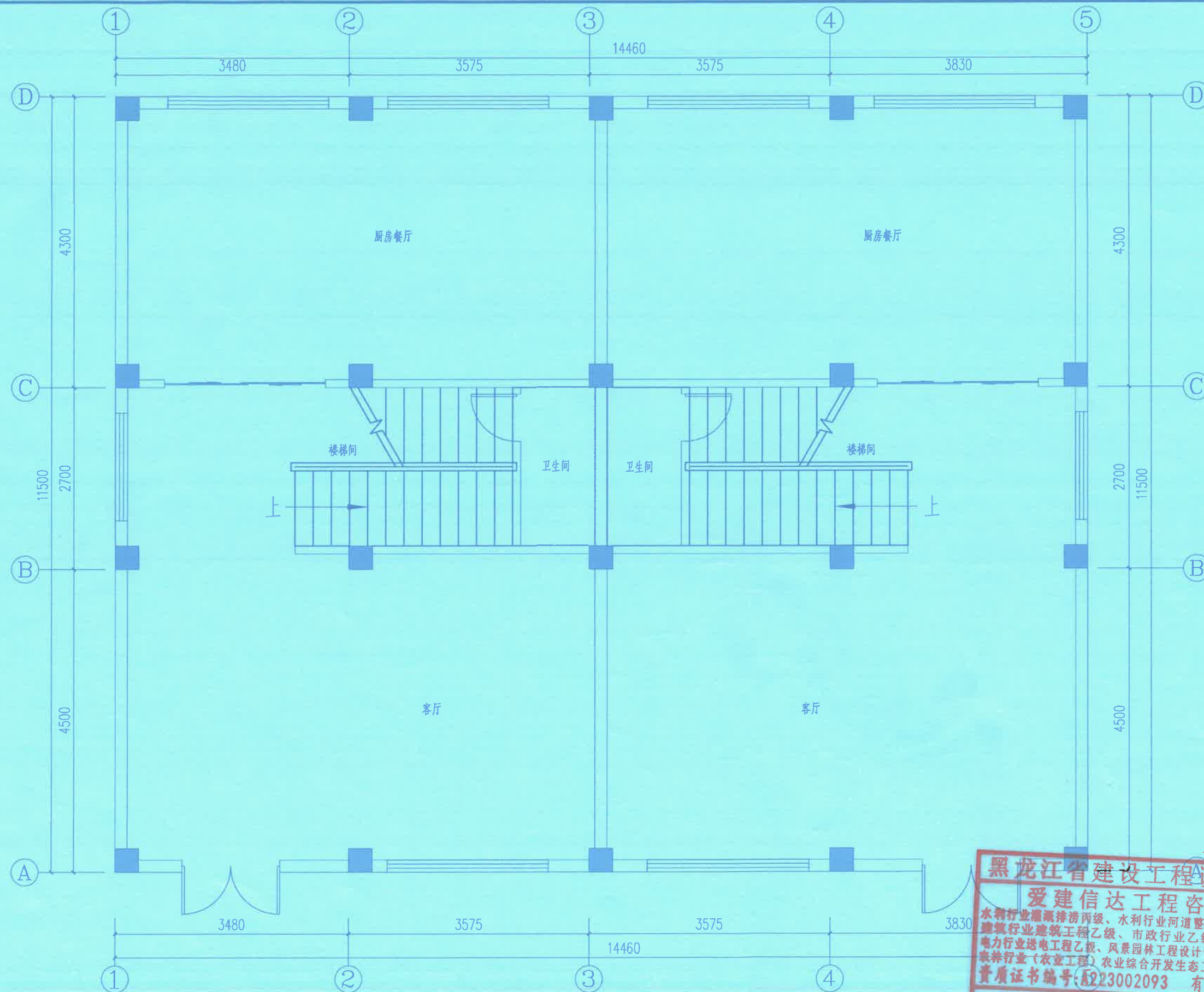
首层平面图 1:100
