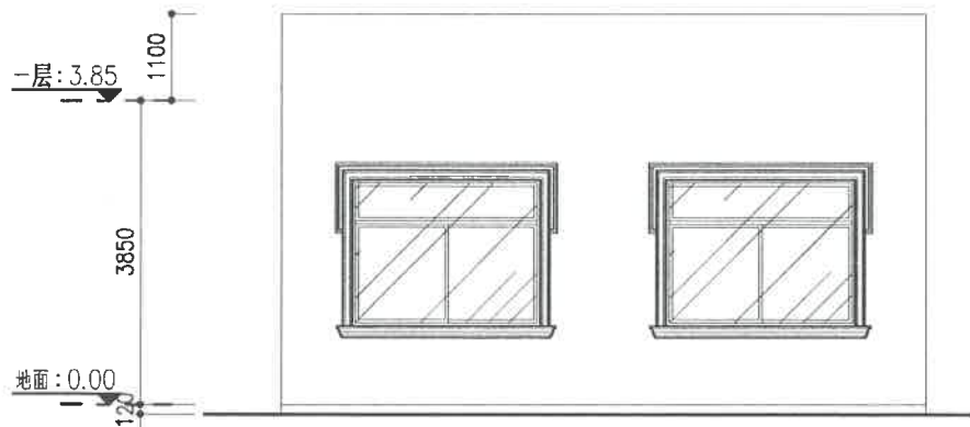
背立面图
