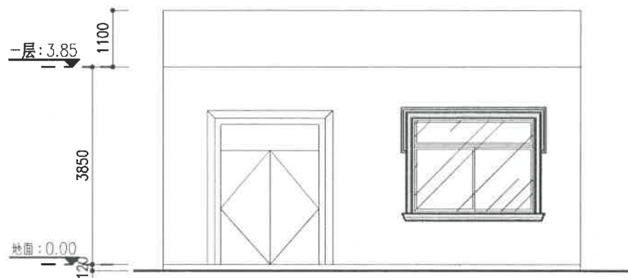
正立面图
