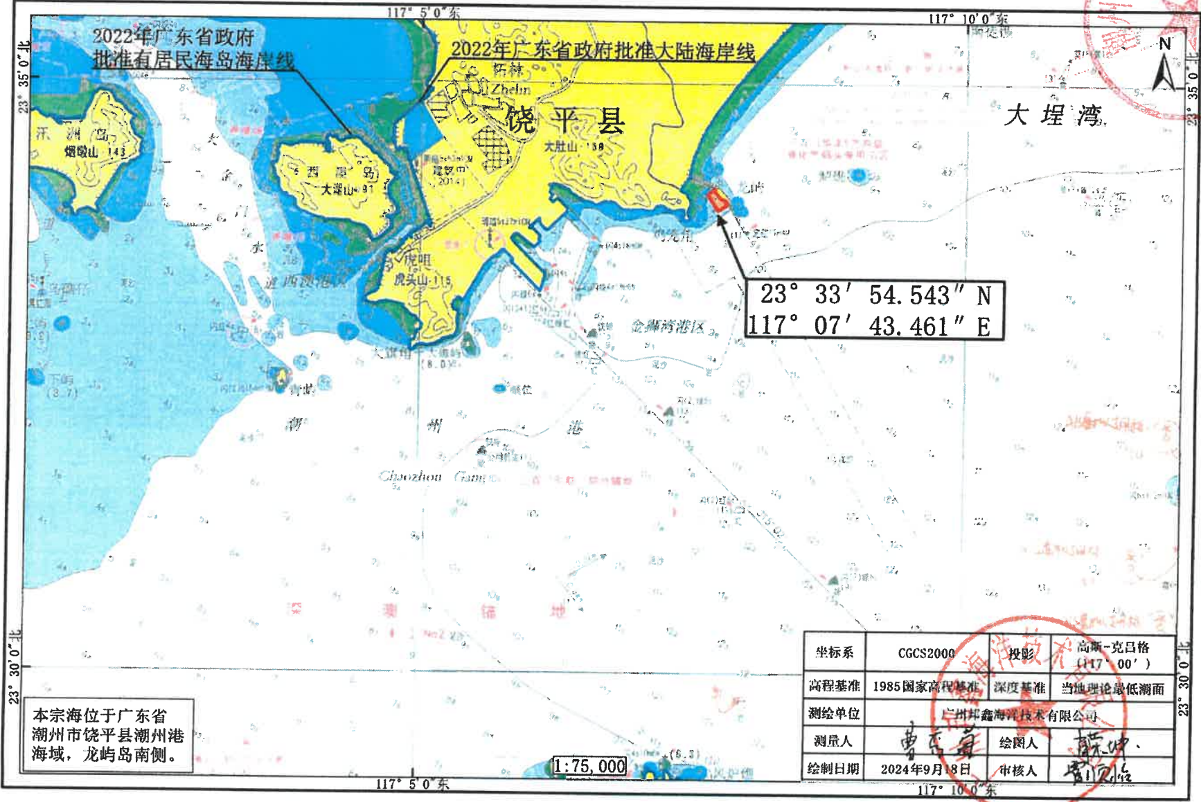
潮州市华丰造气厂有限公司2000吨码头项目（码头、栈桥和港池）用海变更后宗海位置图
