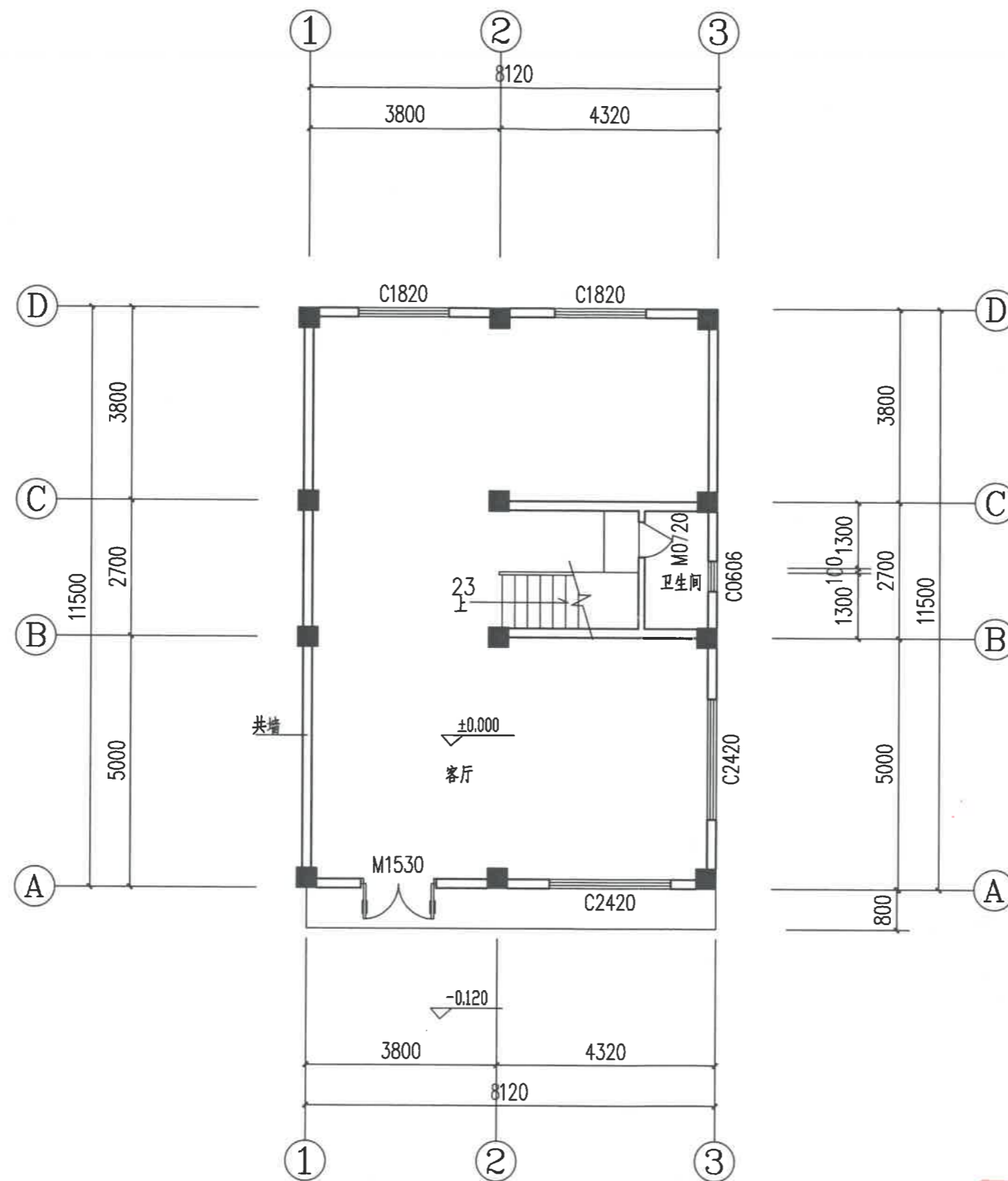
底层平面图 1:100
