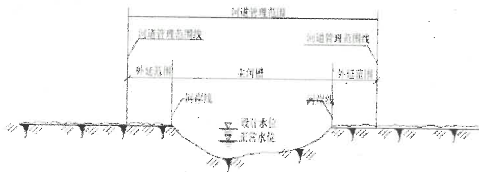
附图 1-2 无堤防平原区河道管理范围示意图
