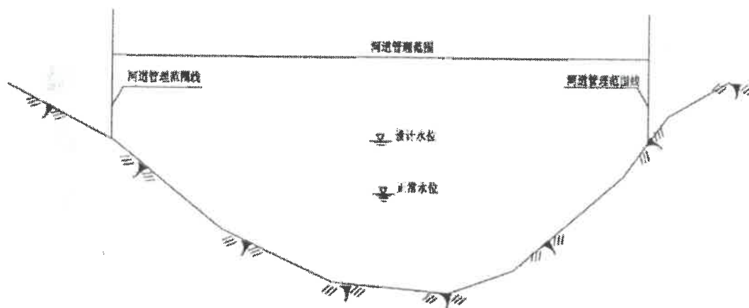
附图 1-3 无堤防山区河道管理范围示意图
